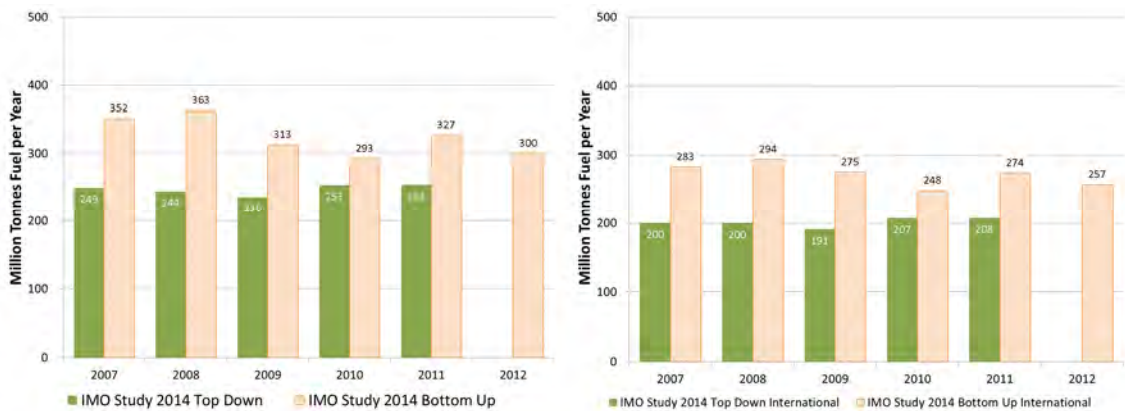
a. All marine fuels
